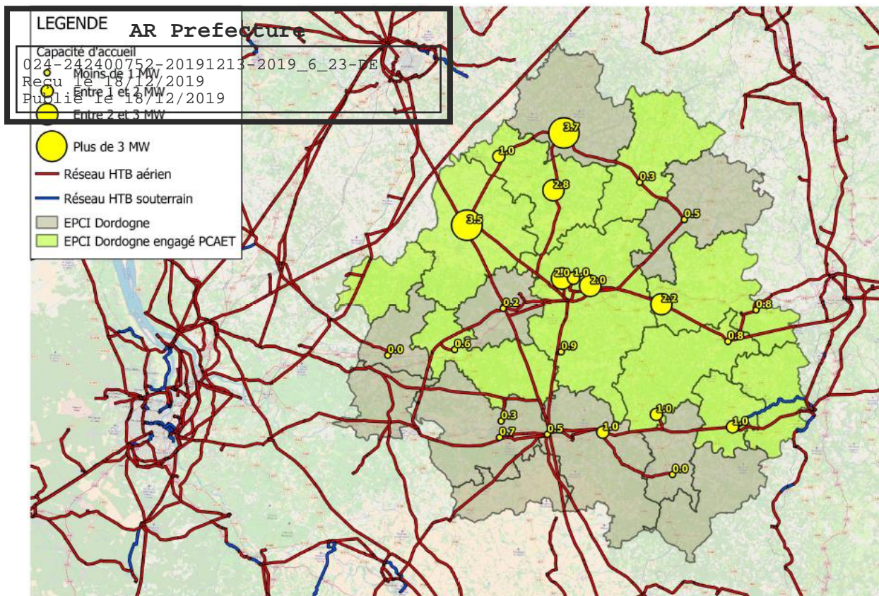
Figure 3. Capacité réservée par poste de transformation HTB/HTA au titre du S3REnR ( source : RTE)
