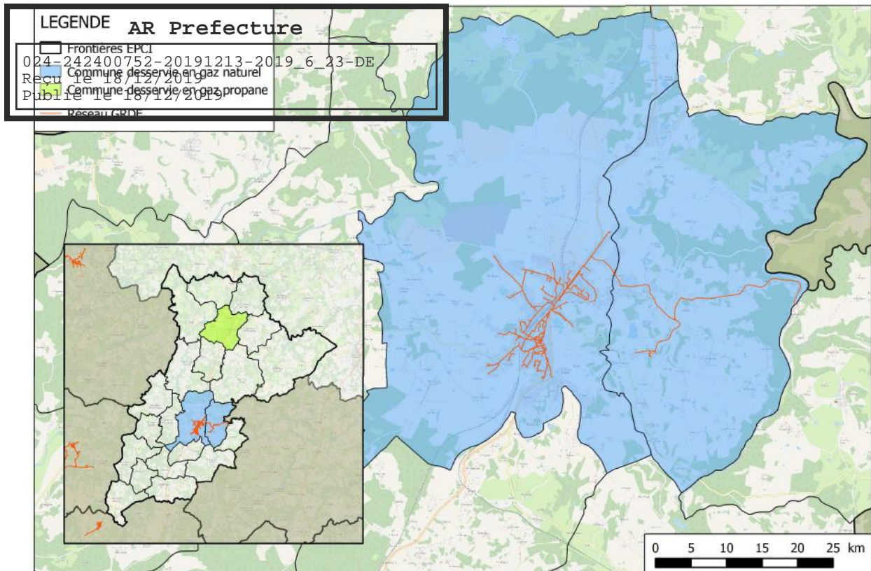
Figure 5. Cartographie des communes desservies en gaz et du réseau de distribution de GRDF (source : SDE 24 et GRDF)
