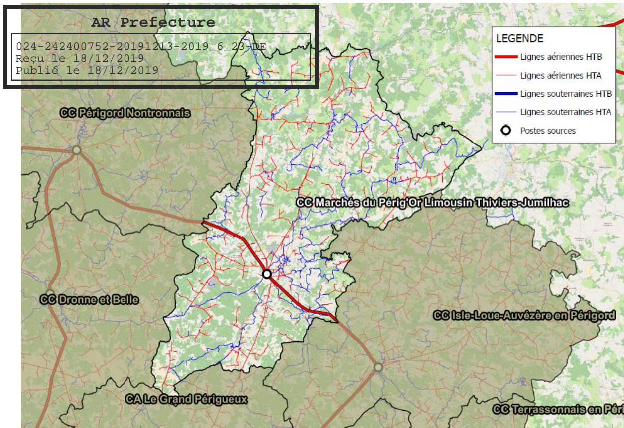
Figure 2. Cartographie des réseaux HTB et HTA sur la CC Périgord-Limousin (source : RTE et Enedis)
